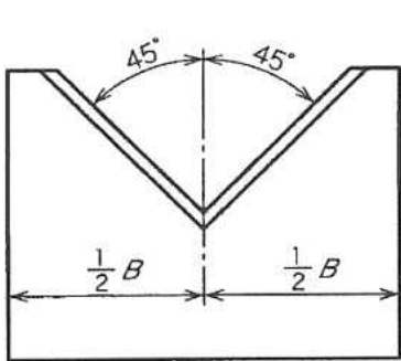
< 직각 삼각 위어 >
