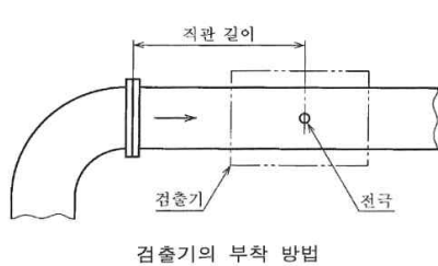
< 배관형 전자 유량계 설치 위치 >
