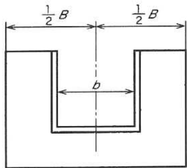
< 사각 위어 >
